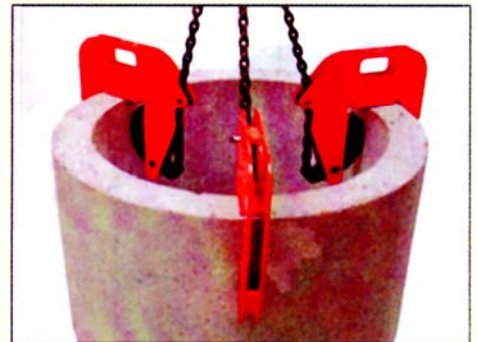
Modèle IPCC
