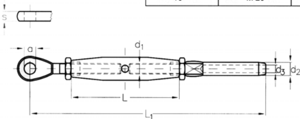
ASS Mini-Ridoir à œil et terminaison simple
