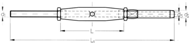
ASS Mini-Ridoir à tige filetée et terminaison simple
