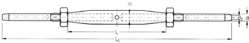
Ridoir INOX à deux terminaisons simples standard
