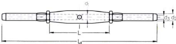
ASS Mini-Ridoir à deux terminaisons simples
