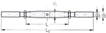
ASS Super-Mini-Ridoir à deux terminaisons simples
