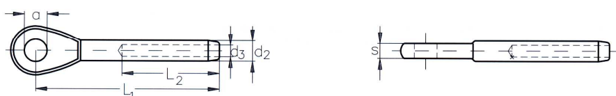
ASS Mini-Terminaison à œil
