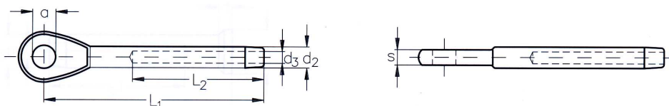
Terminaison à œil INOX standard
