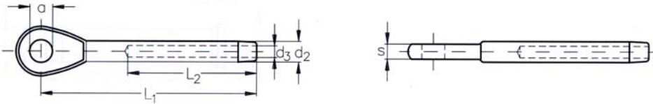
Terminaison à œil INOX standard
