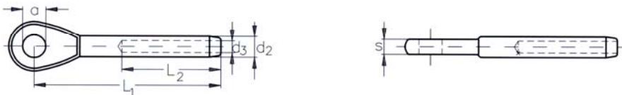
ASS Mini-Terminaison à œil
