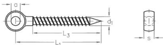
Vis à œil INOX, DIN 447 filetage bois à droite
